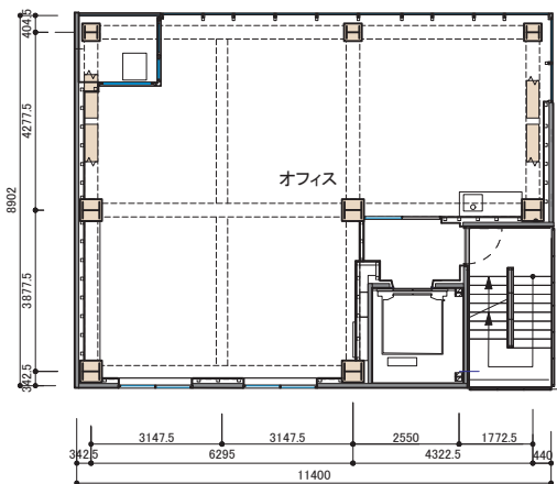
5階平面図 1:200
