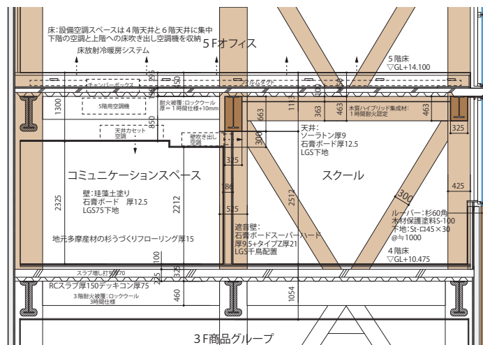
断面詳細図 1:100
